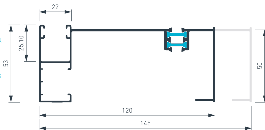
HSL-A-120 Thermal Break # 027242
