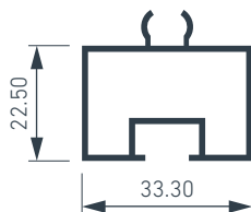
Fly Screen Ext. PVC 33x22,5
